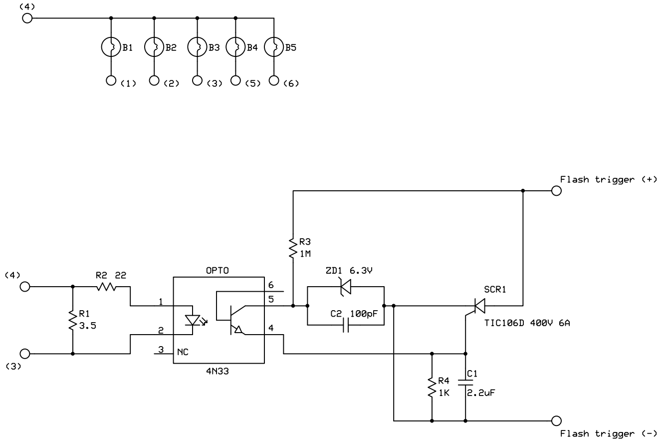
Flashbar wiring
